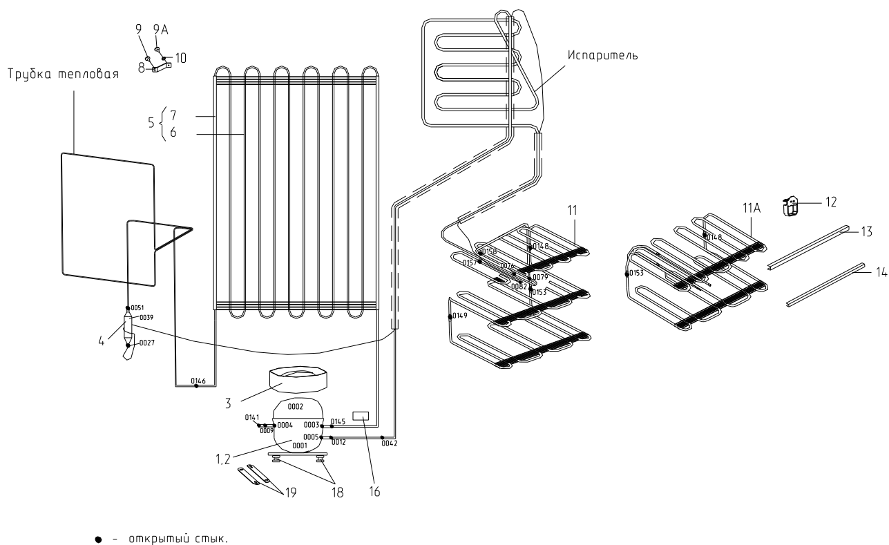
Рисунок 6 - Схема холодильного агрегата ( компрессор типа DLX )
