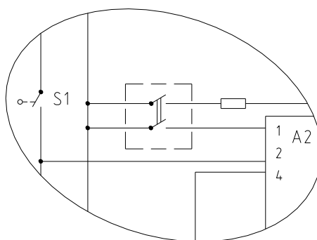
Рисунок А.3 - Схема электрическая принципиальная
