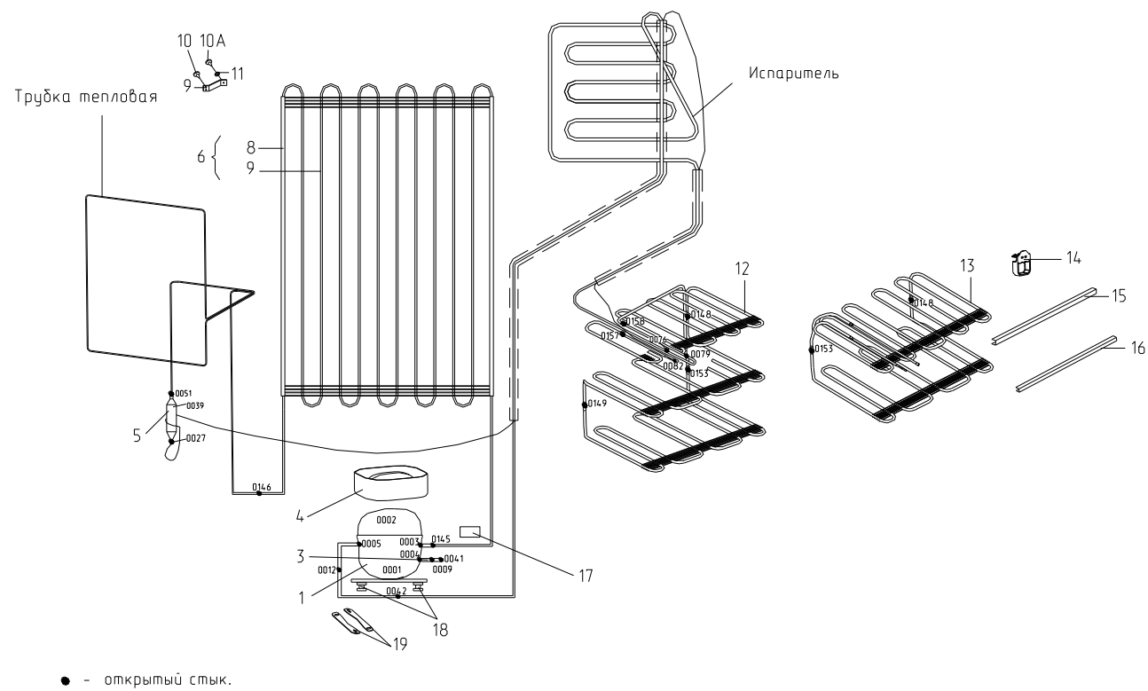
Рисунок 5 - Схема холодильного агрегата (компрессор типа CTB, CTC, TLY)
